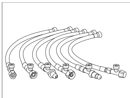
Fig. 249 Mangueras de alta presión con dispositivo de seguridad en caso de rotura de manguera (variantes país específicas)
