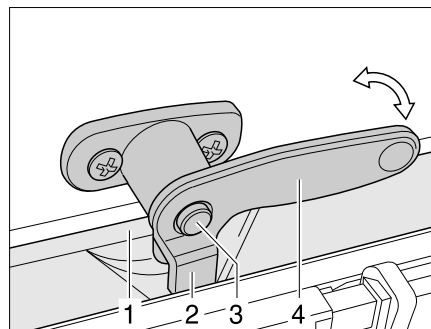
Fig. 76 Palanca de bloqueo con botón de seguridad en posición "cerrado"
