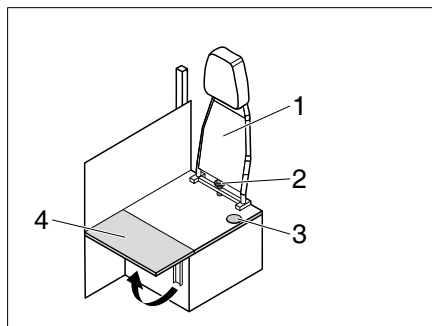
Fig. 214 Transformación del funcionamiento con el vehículo en marcha al funcionamiento para vivir y estar
