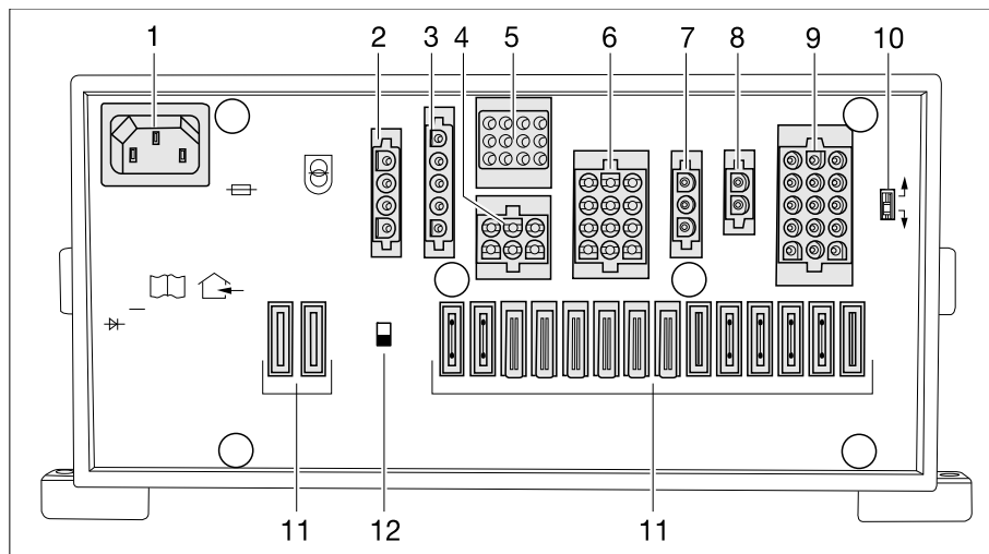
Fig. 255 Bloque eléctrico (EBL 119)
