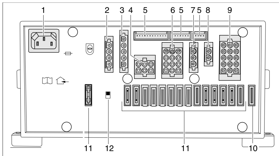
Fig. 254 Bloque eléctrico (EBL 111)
