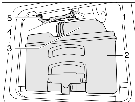
Fig. 373 Tubo de desagüe del depósito de agua del inodoro
