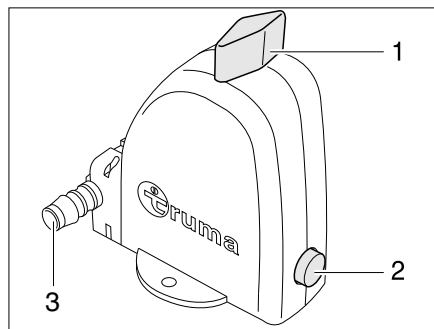
Fig. 321 Válvula de seguridad/purga de la caldera - Posición de funcionamiento
