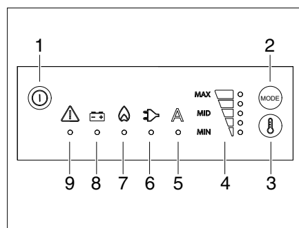
Fig. 336 Elementos de mando para el frigorífico (Dometic de la serie 10, modelo RM 10.5)
