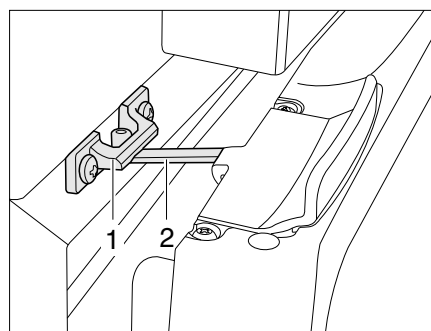
Fig. 343 Puerta del frigorífico en posición de ventilación (Thetford)
